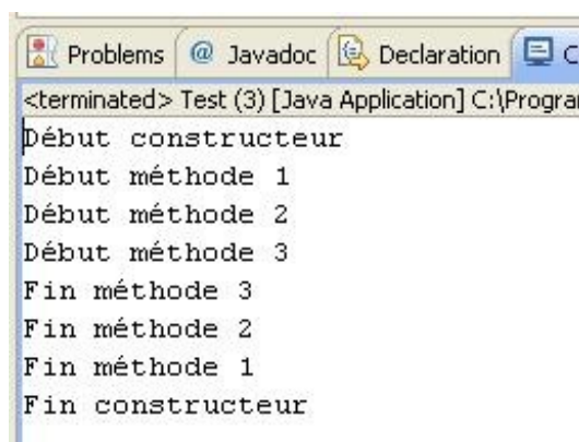
Exemple de pile d'invocations
