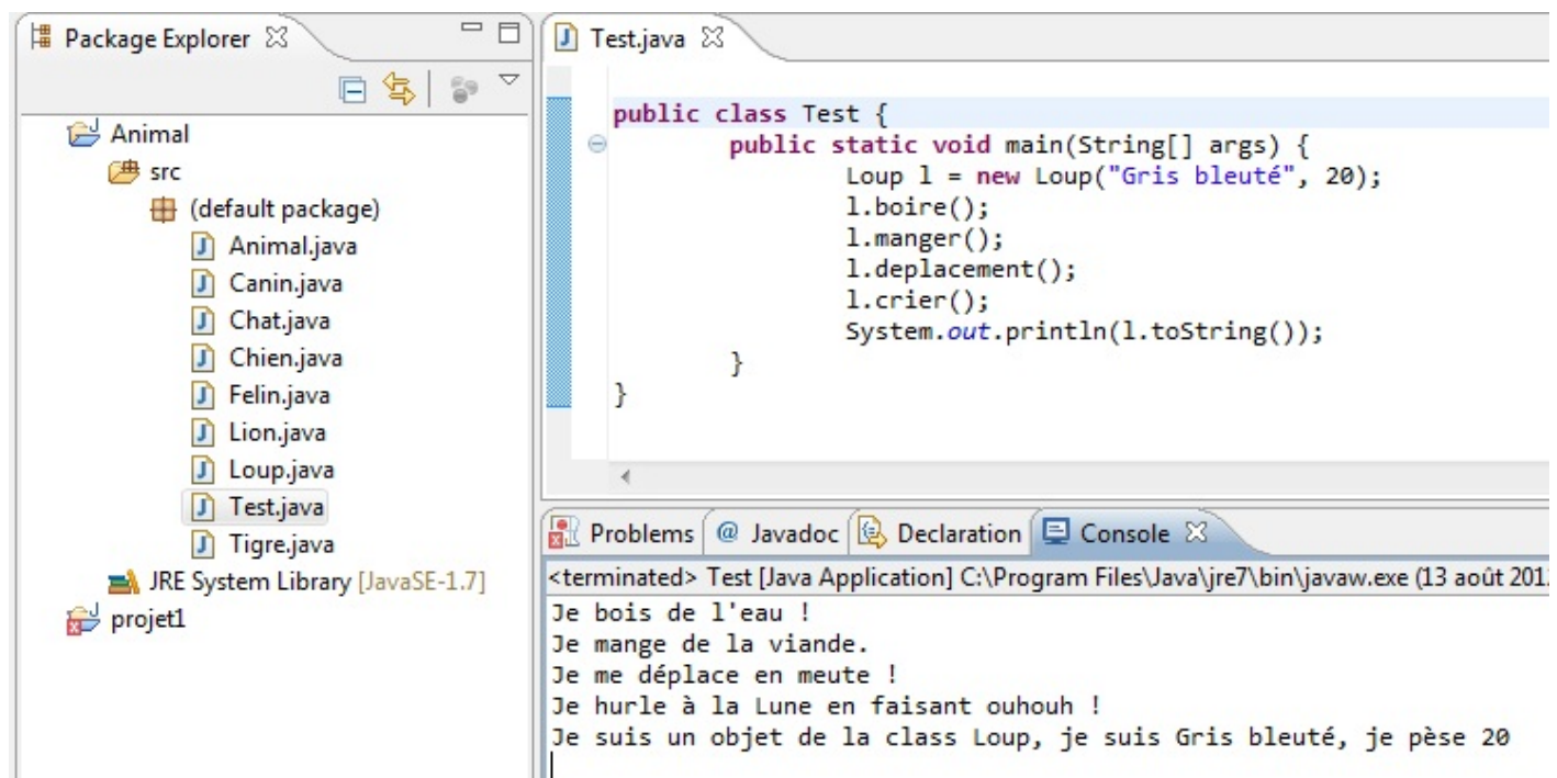
Test d'une classe abstraite
