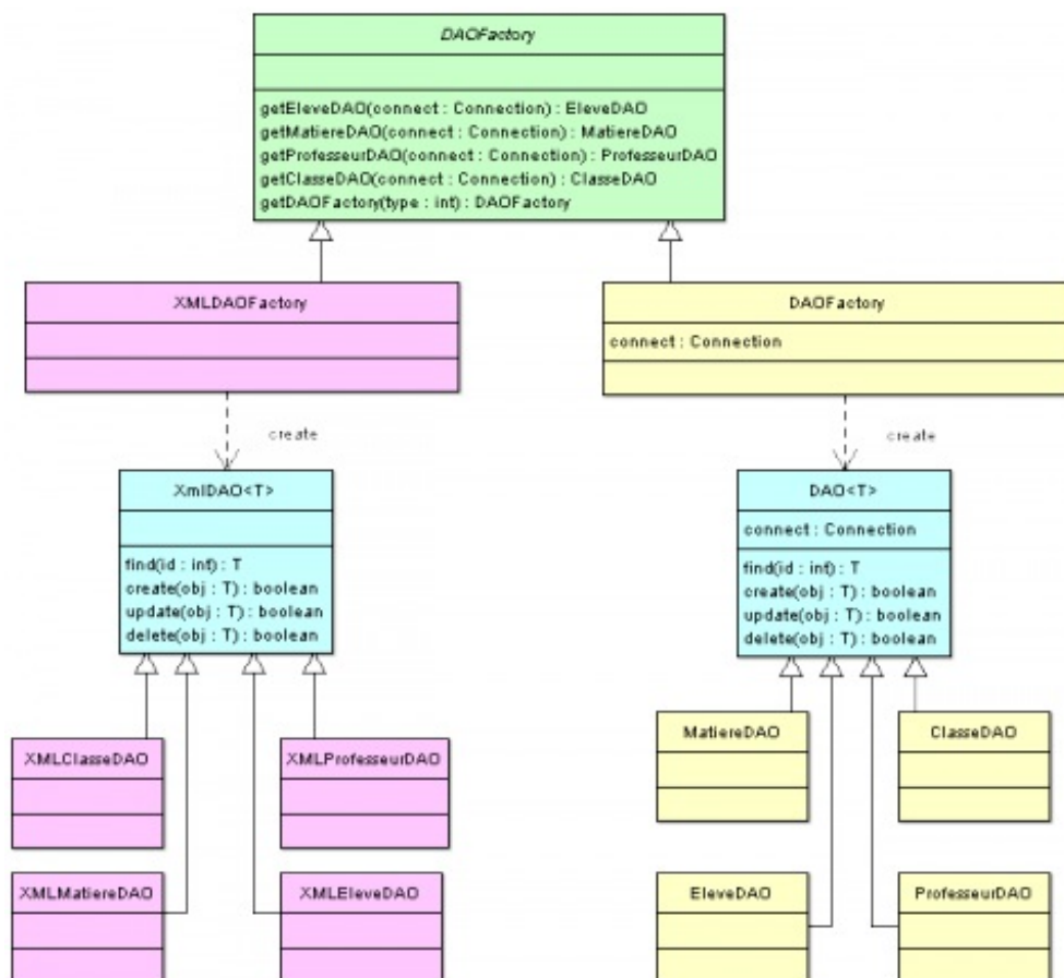
Diagramme de classe de nos factory
