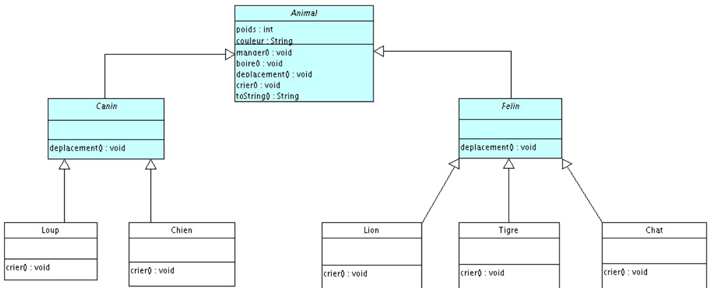
Nouvelle architecture des classes
