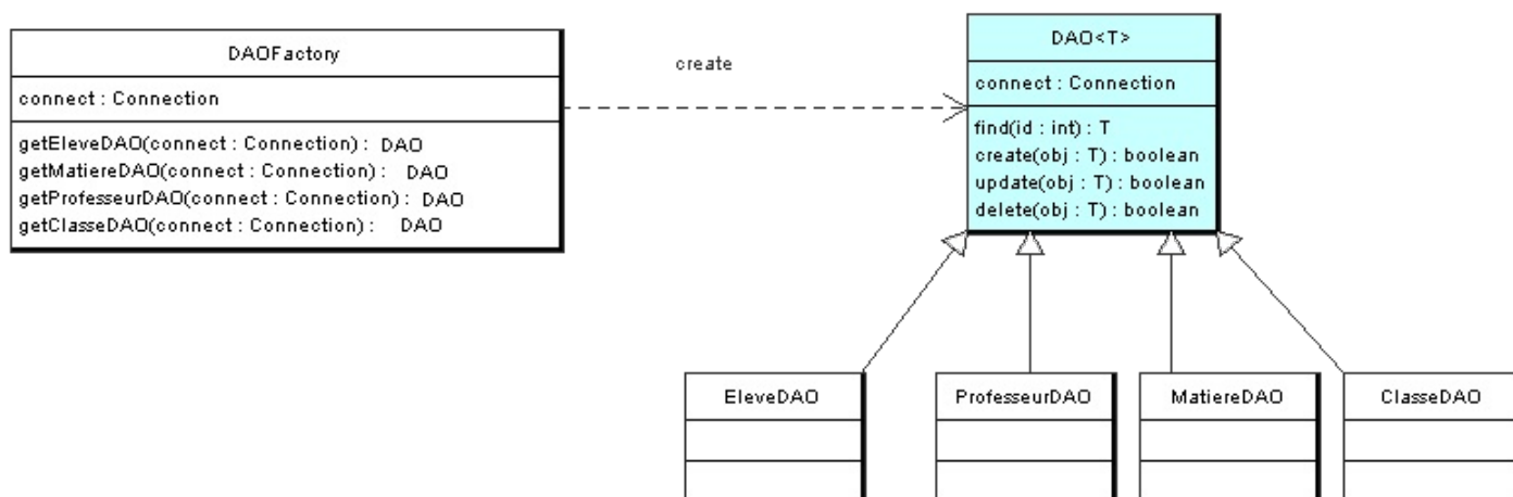
Diagramme de classe de notre fabrique
