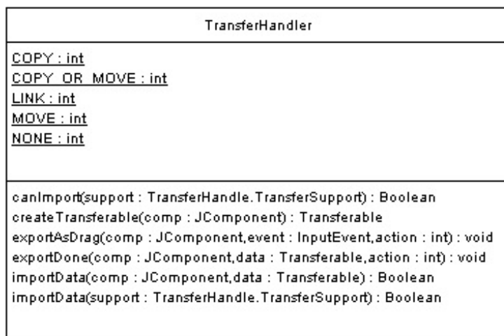
La classe TransferHandler
