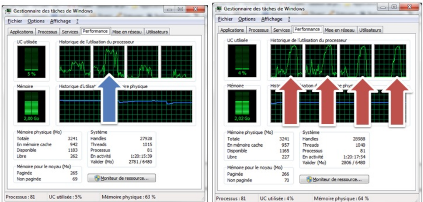
À gauche en mode normal, à droite en mode Fork/Join
