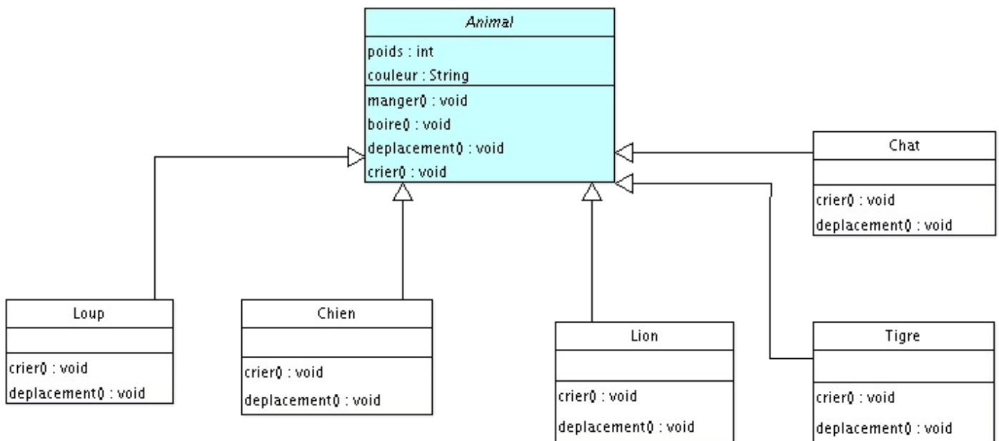
Hiérarchie de nos classes
