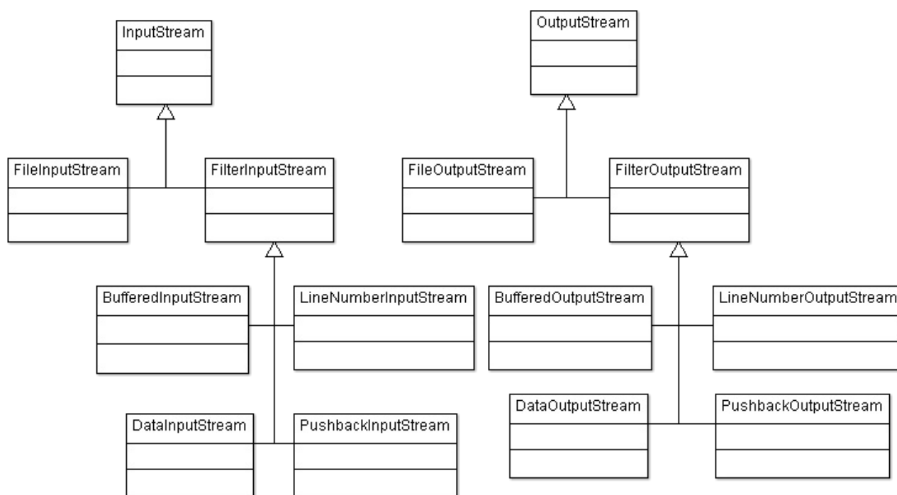
Hiérarchie des classes du package java.io
